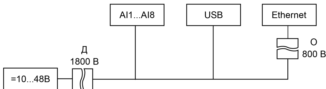
Рисунок 2.1 – Изоляция узлов прибора
